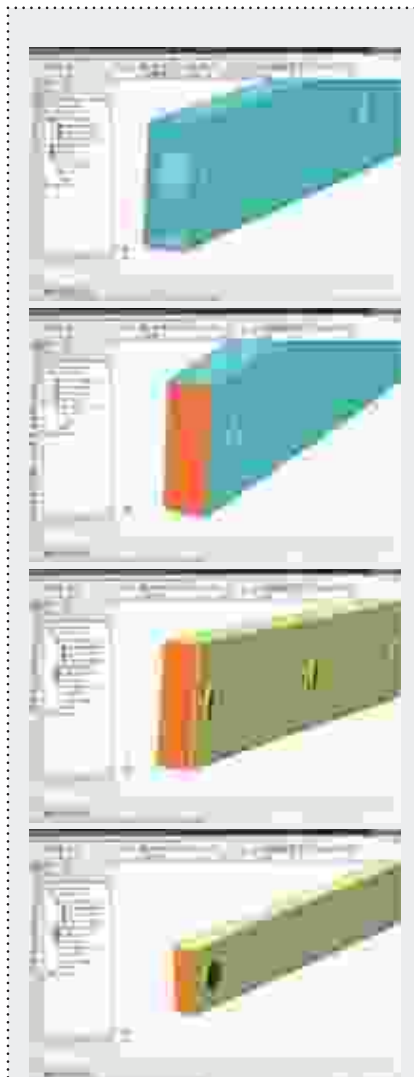
↑ Рис. 3. Создание детали «заглушка» в контексте сборочной модели балки подъемника с последующим изменением размеров балки
